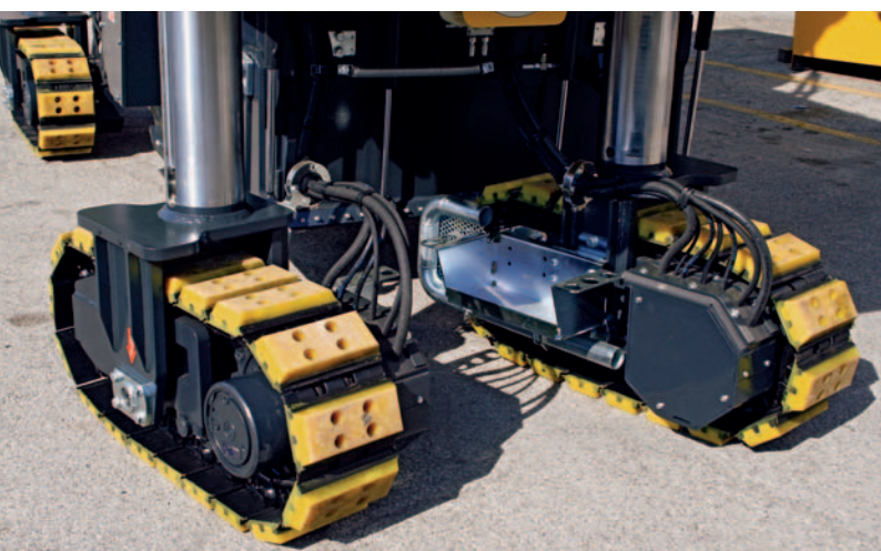
Улучшенные гусеницы.
